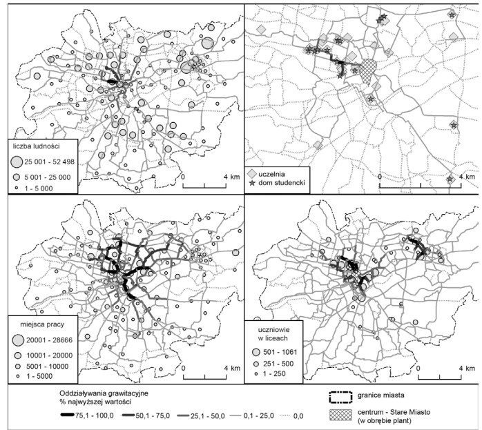
Rys. 2. Oddziaływania grawitacyjne
