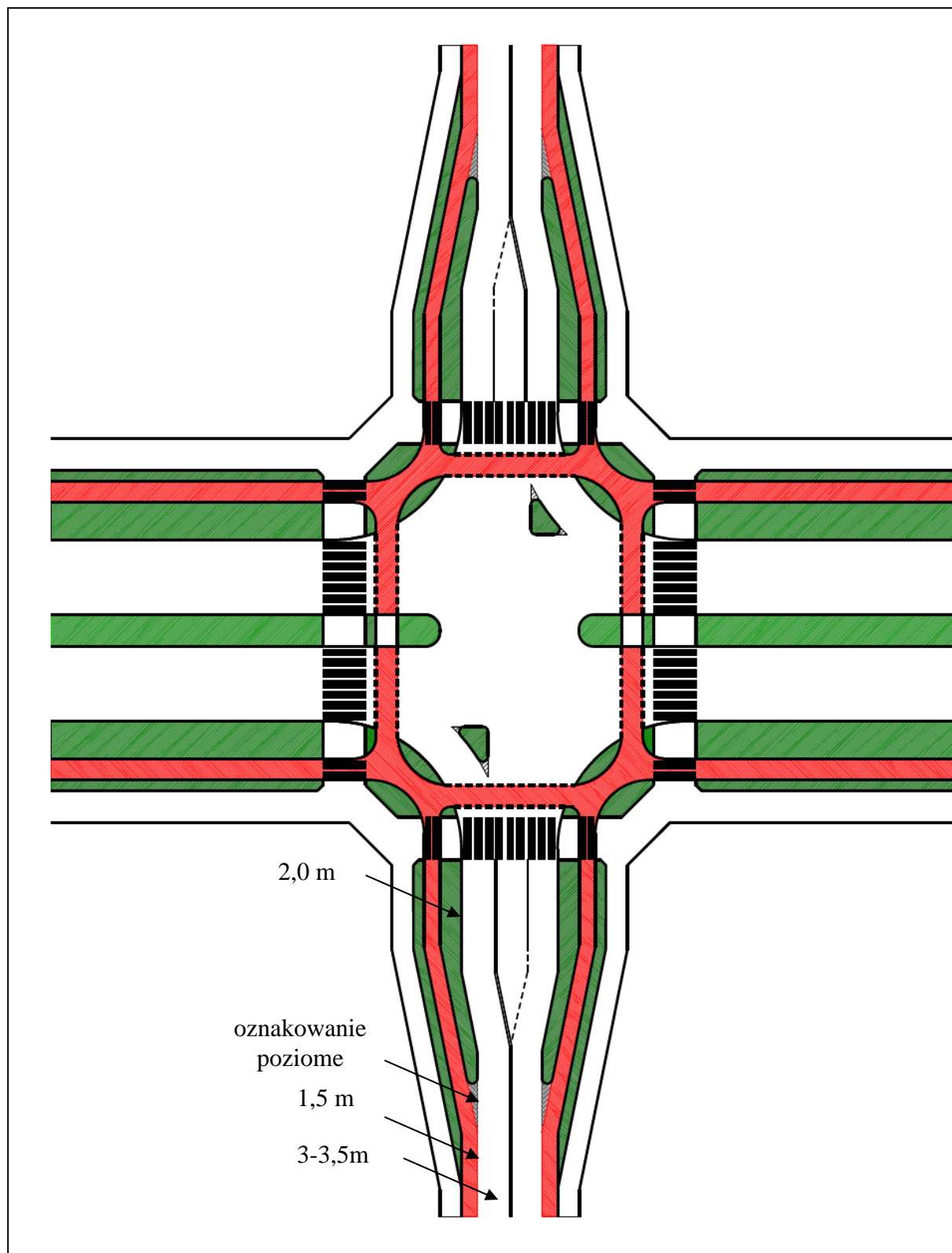
Rys. 15 Przykład rozwiązania skrzyżowania drogi nadrzędnej i podporządkowanej z ruchem rowerowym prowadzonym na pasach dla rowerów.
